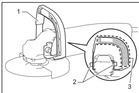
► 1. Mango cuadrado 2. Tornillo 3. Empuñadura
