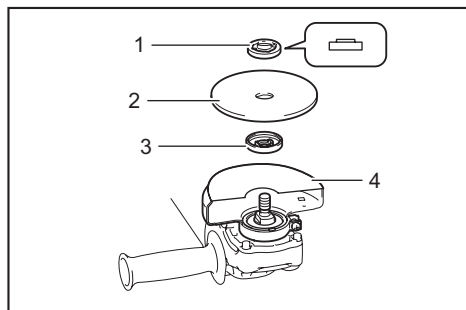
► 1. Contre-écrou 2. Meule tronçonneuse abrasive / meule diamant 3. Flasque intérieur 4. Protecteur de meule pour meule tronçonneuse abrasive / meule diamant
